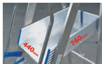
PIATTAFORMA DI LAVORO MM 760X440 IN LAMIERA MANDORLATA DI ALLUMINIO CON TAVOLE FERMAPIEDE Workplatform 760x440 mm in grooved aluminum sheet, with toabords
